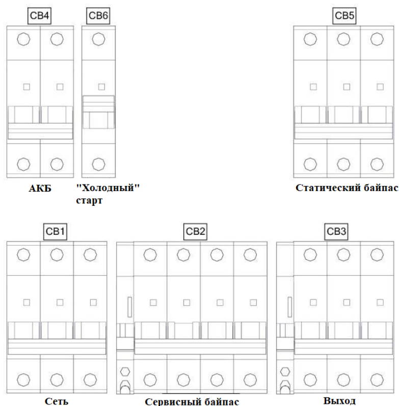
Рисунок 3.2. Автоматические выключатели
