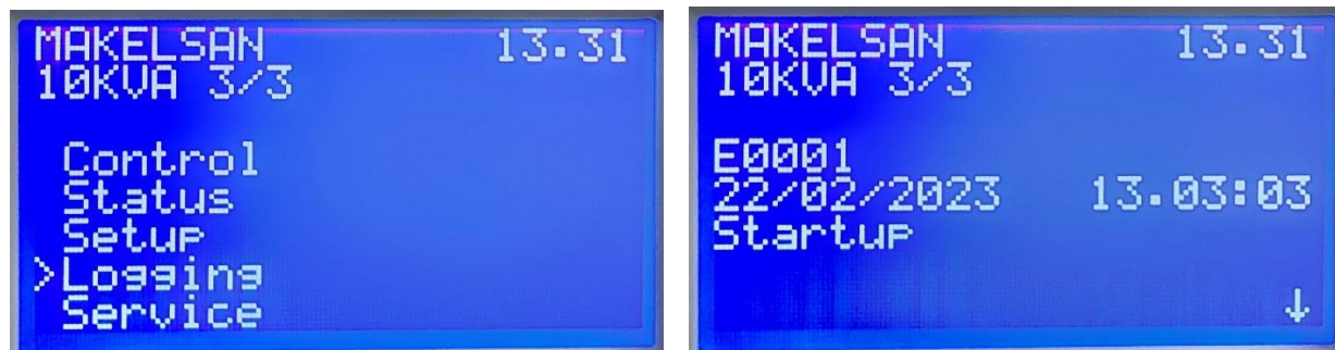
Рисунок 2.31. Журнал событий
